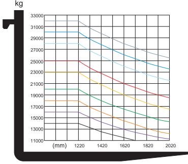
Yük Grafiği/ Load Chart Kaldırma Yüksekliği/ Lift Height ≤ 4500 mm
