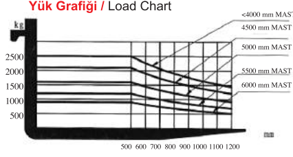
2.5 T Yük Grafiği / Load Chart
